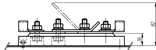
E 端子 (1/3)
