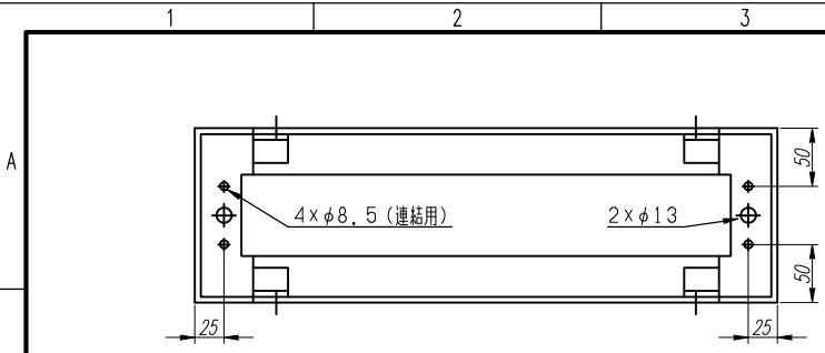
イ-イ视图
