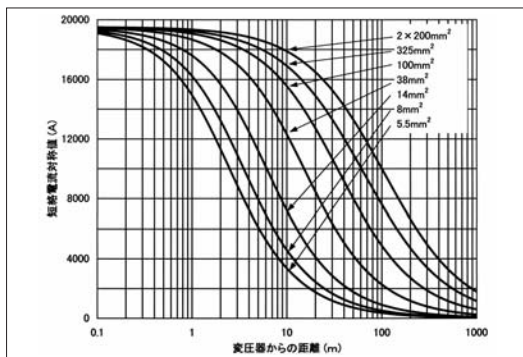
図1.5 3φ3W変圧器容量 200kVA 二次電圧 210V
