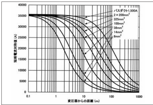
図1.7 3 \phi 3W変圧器容量 500kVA 二次電圧 210V
