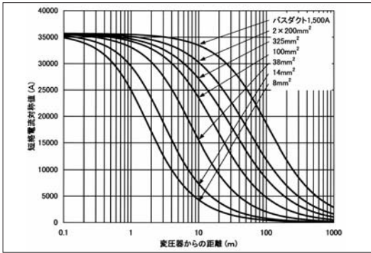
図2.9 1φ3W変圧器容量 300kVA 外線間 210V
