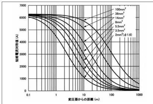
図1.1 3φ3W変圧器容量 50kVA 二次電圧 210V
