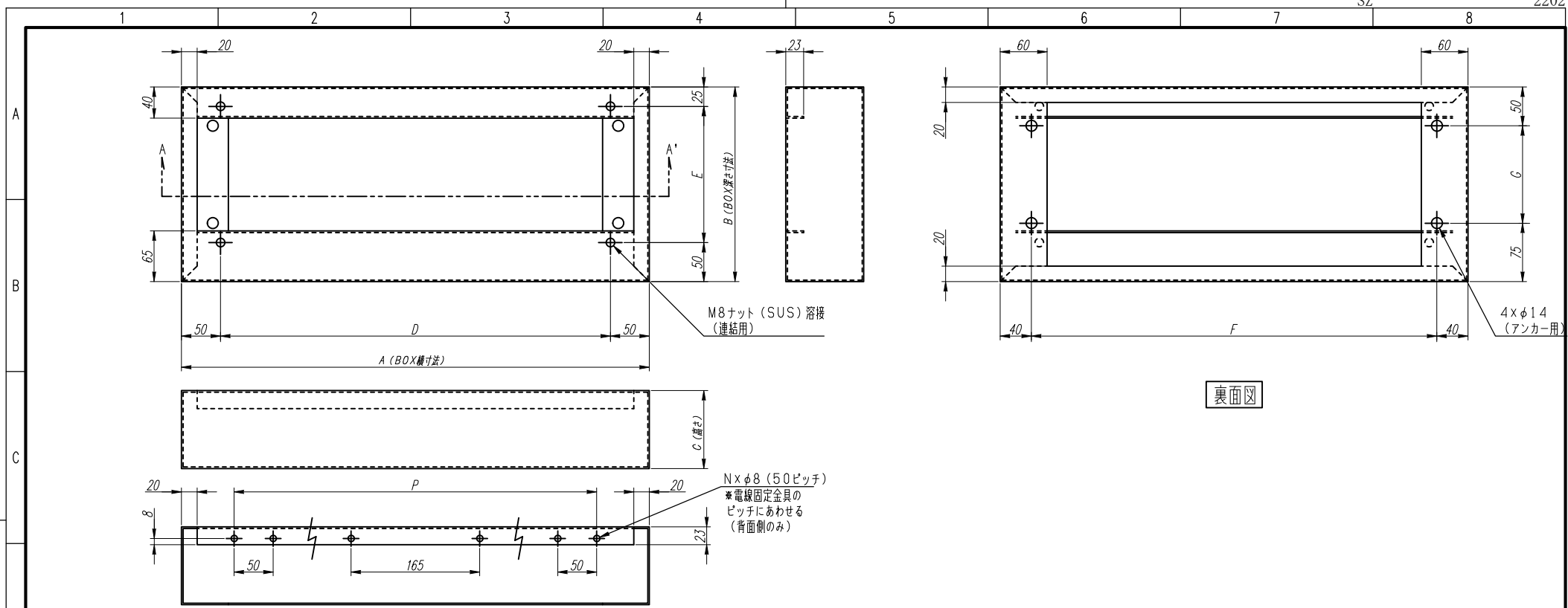
A-A' 矢視図
