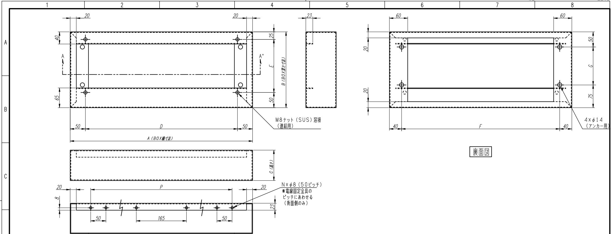
A-A' 矢視図
