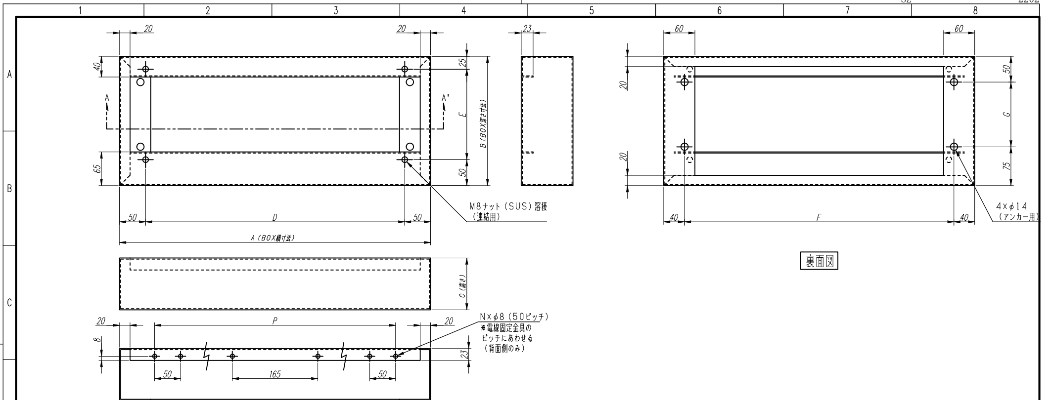
A-A' 矢視図
