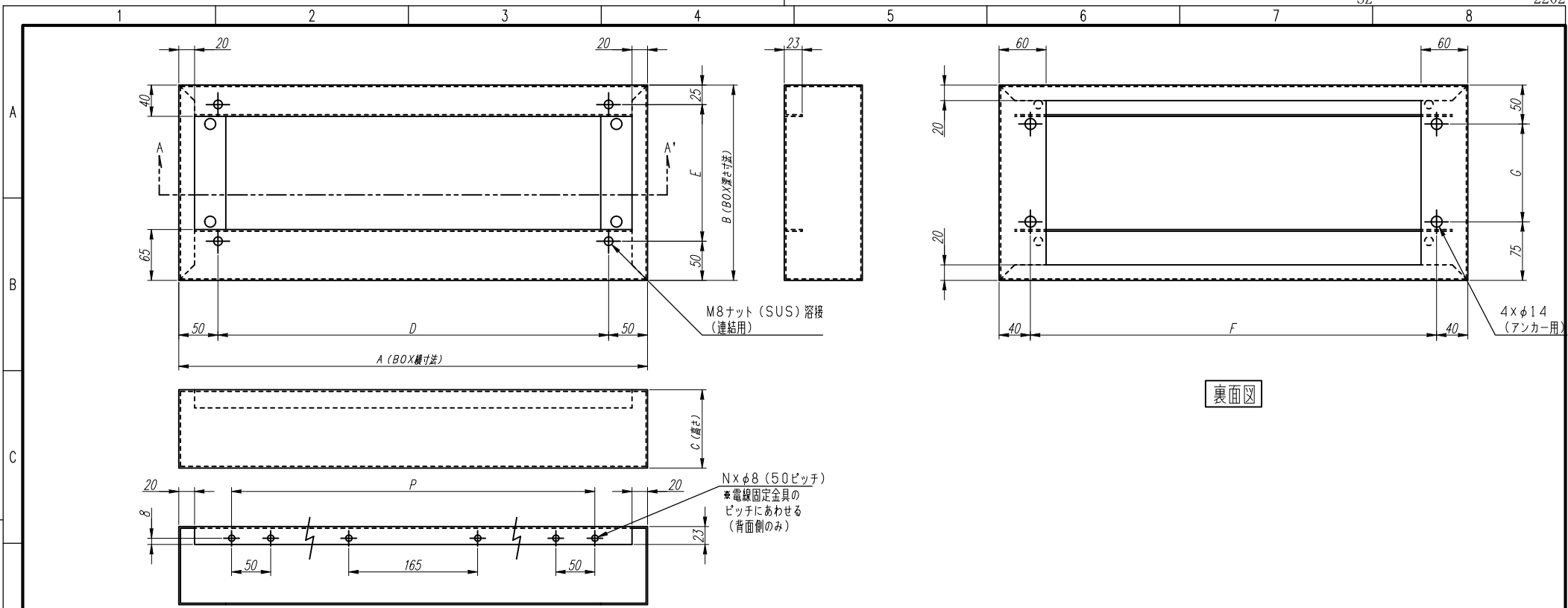
A-A' 矢視図
