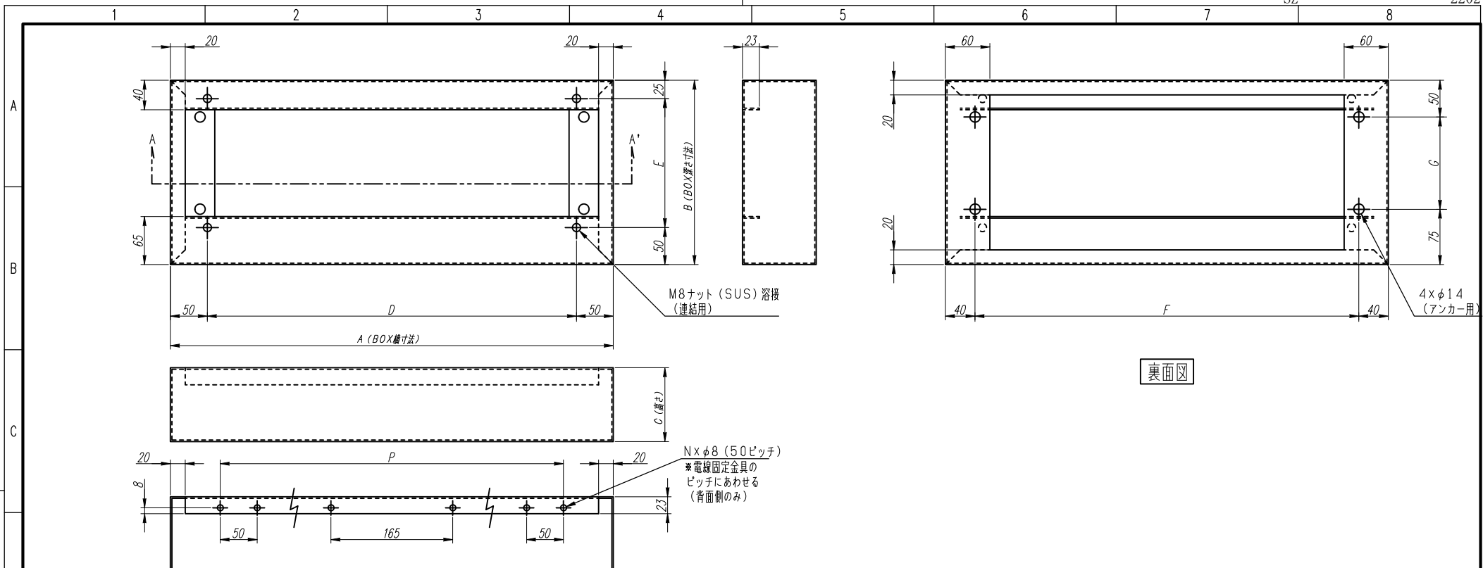
A-A' 矢視図
