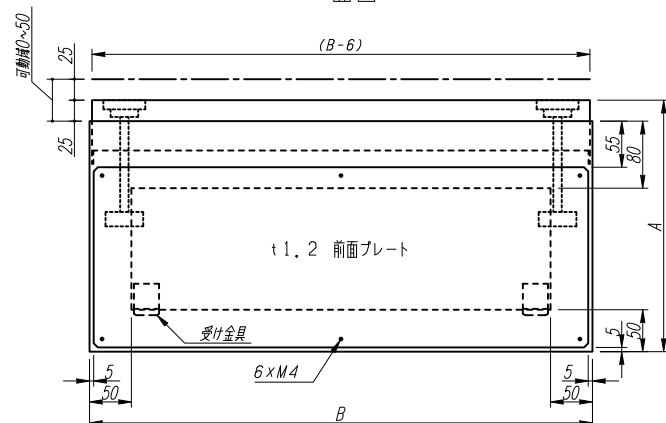
正面图
