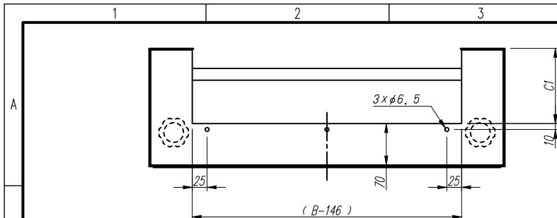
上面图
