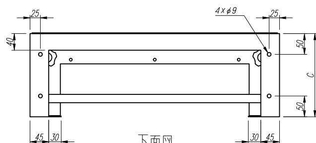
下面图
