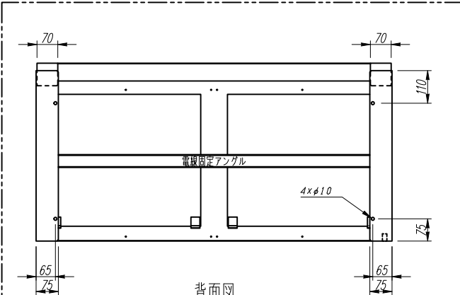
背面図
