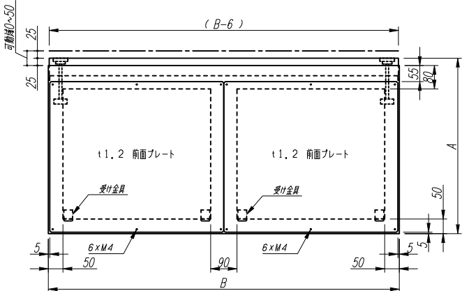
正面図
