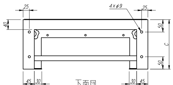
下面図
