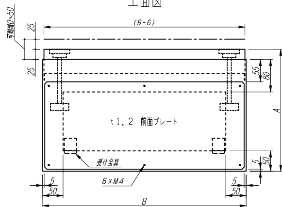
正面図
