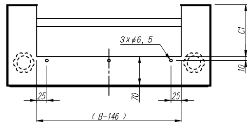
上面図
