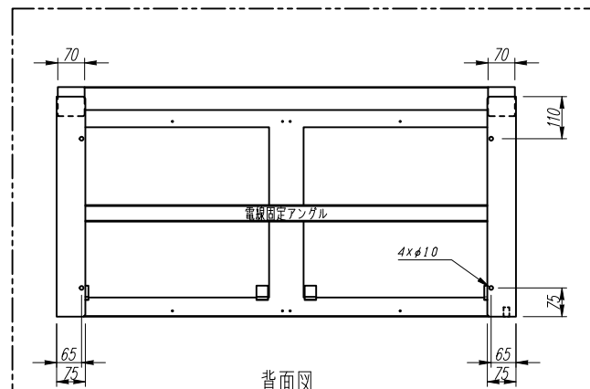
背面図
