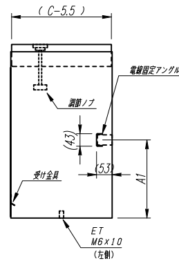
側面図
