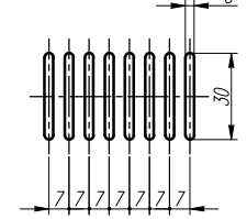
スリット部詳細図 (縮尺1/2) 3
