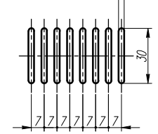
スリット部詳細図 (縮尺1/2) 3
