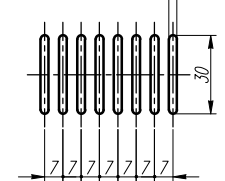
スリット部詳細図 (縮尺1/2) \beta
