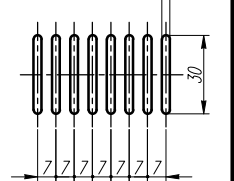
スリット部詳細図 (縮尺1/2) 3
