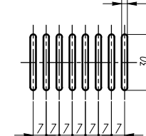
スリット部詳細図 (縮尺1/2) 3
