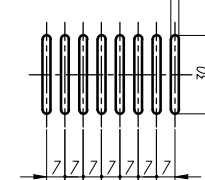
スリット部詳細図 (縮尺1/2) 3
