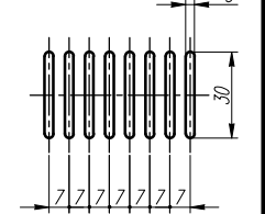
スリット部詳細図 (縮尺1/2) 3
