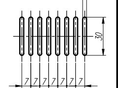
スリット部詳細図 (縮尺1/2) 3
