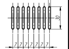
スリット部詳細図 (縮尺1/2) 3
