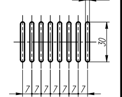
スリット部詳細図 (縮尺1/2) 3
