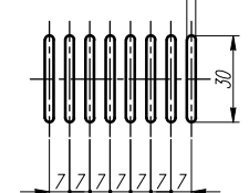
スリット部詳細図 (縮尺1/2) \beta
