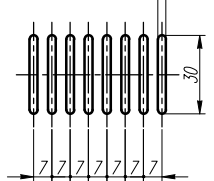
スリット部詳細図 (縮尺1/2) 3
